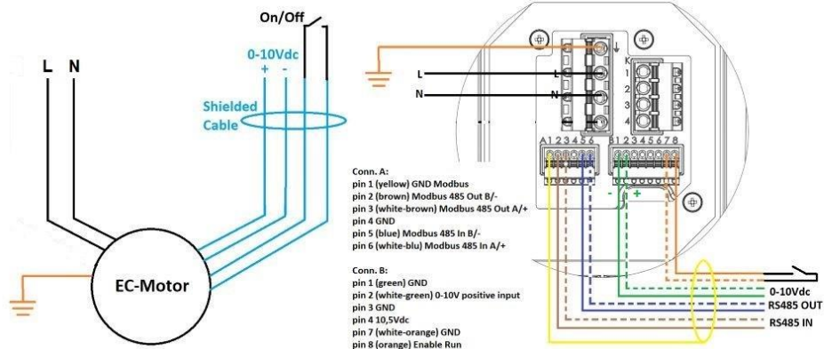
fig.3 schéma de câblage pour les modèles monophasés
