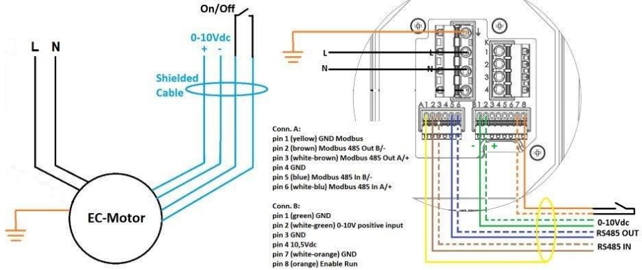
Abb.3 Schaltplan für einphasige Modelle
