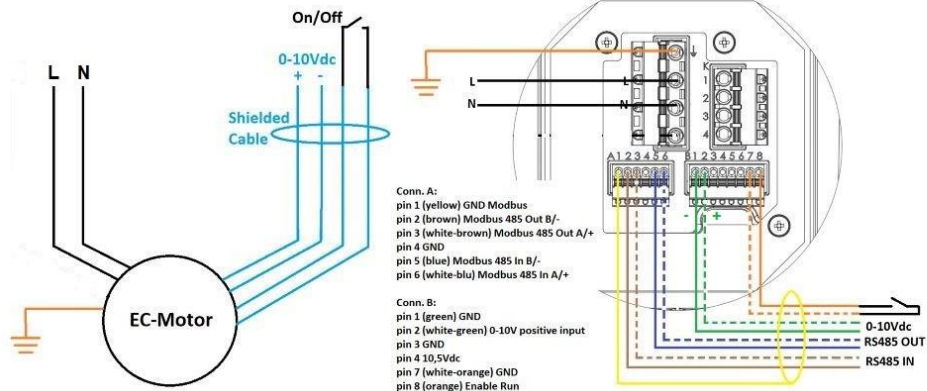
fig.3 diagrama de cableado para modelos monofásicos
