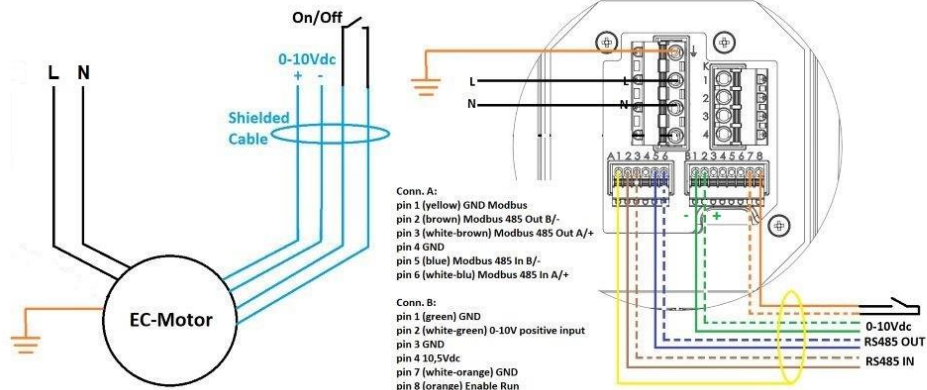
fig.3 schema elettrico modelli monofase
