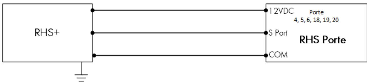
Figur 20: Ledningsdiagram for RHS+-sensor
