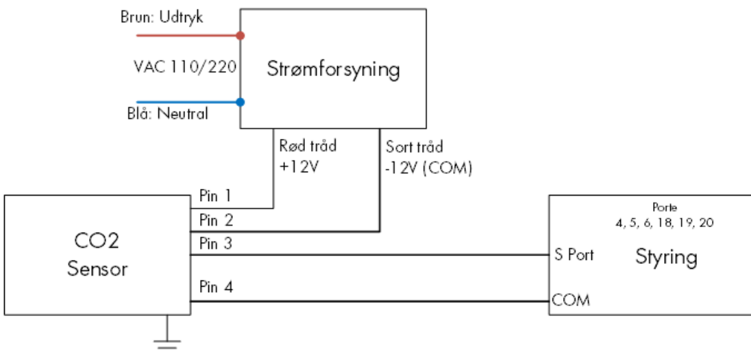
Figur 14: Ledningsdiagram for CO2-sensor
