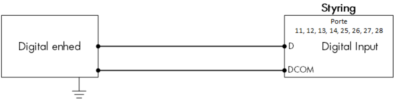
Figur 12: Ledningsdiagram for digitale enheder
