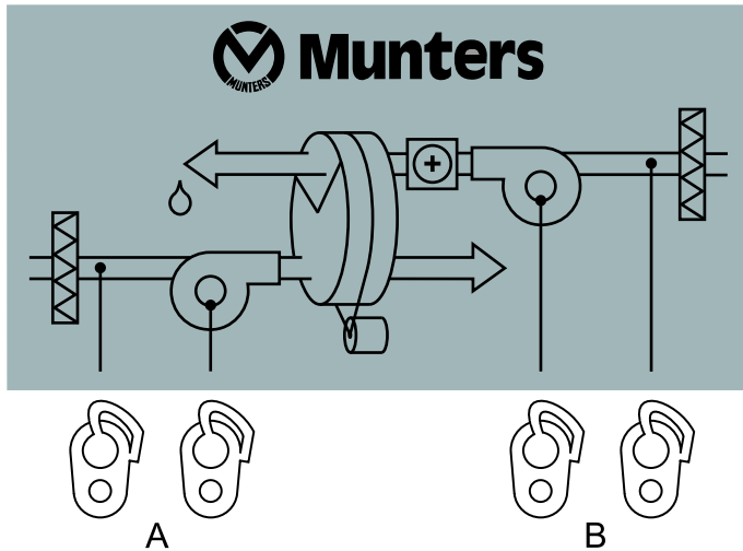
Abb 5.2 Prüfpunkte für Prozess- (A) und Regenerationsluftstrom (B)
