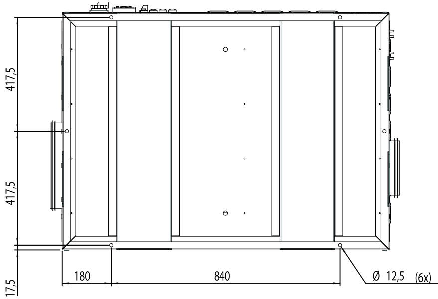
Abb 4.1 Grundrahmen
