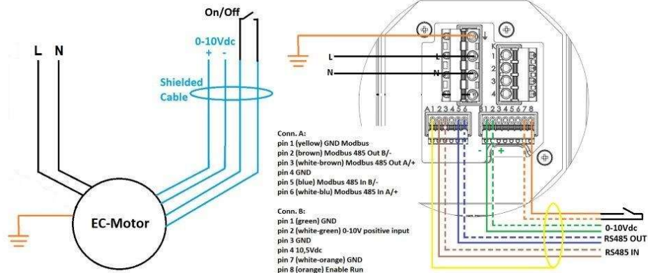
fig.3 schéma de câblage pour les modèles monophasés
