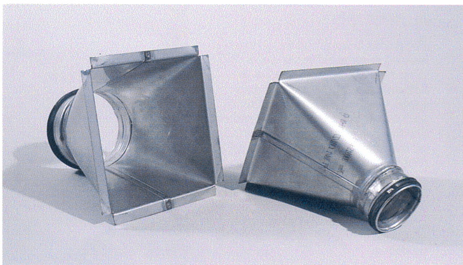
Overgangsstykker for regenereringsluft og procesluftindtag
