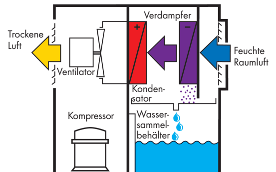
Kälte-Luftentfeuchter
