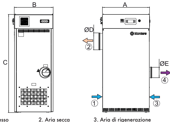
1. Aria di processo 2. Aria secca 3. Aria di rigenerazione 4. Aria umida
