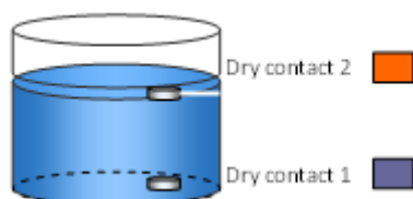
Serbatoio d'acqua con galleggianti
