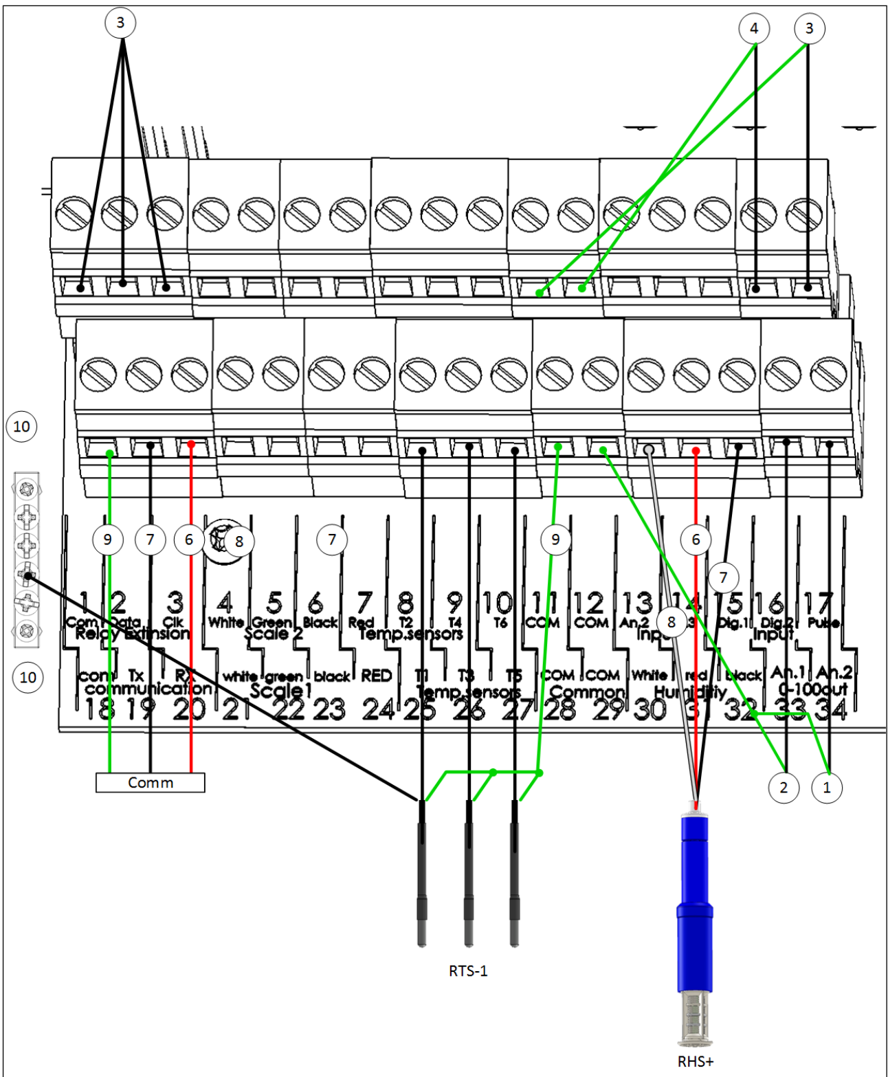
Figura 5: AC-2000 Plus Cableado Eléctrico de Baja Tensión
