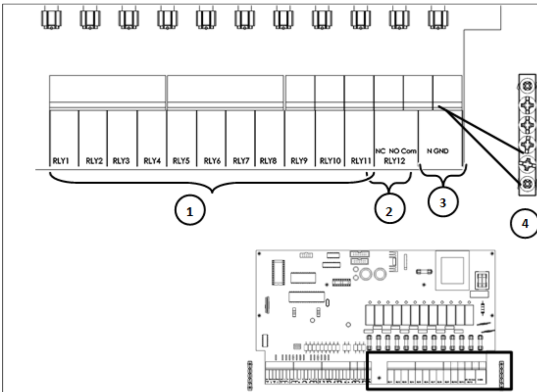
Figura 7: AC-2000 SE Relés
