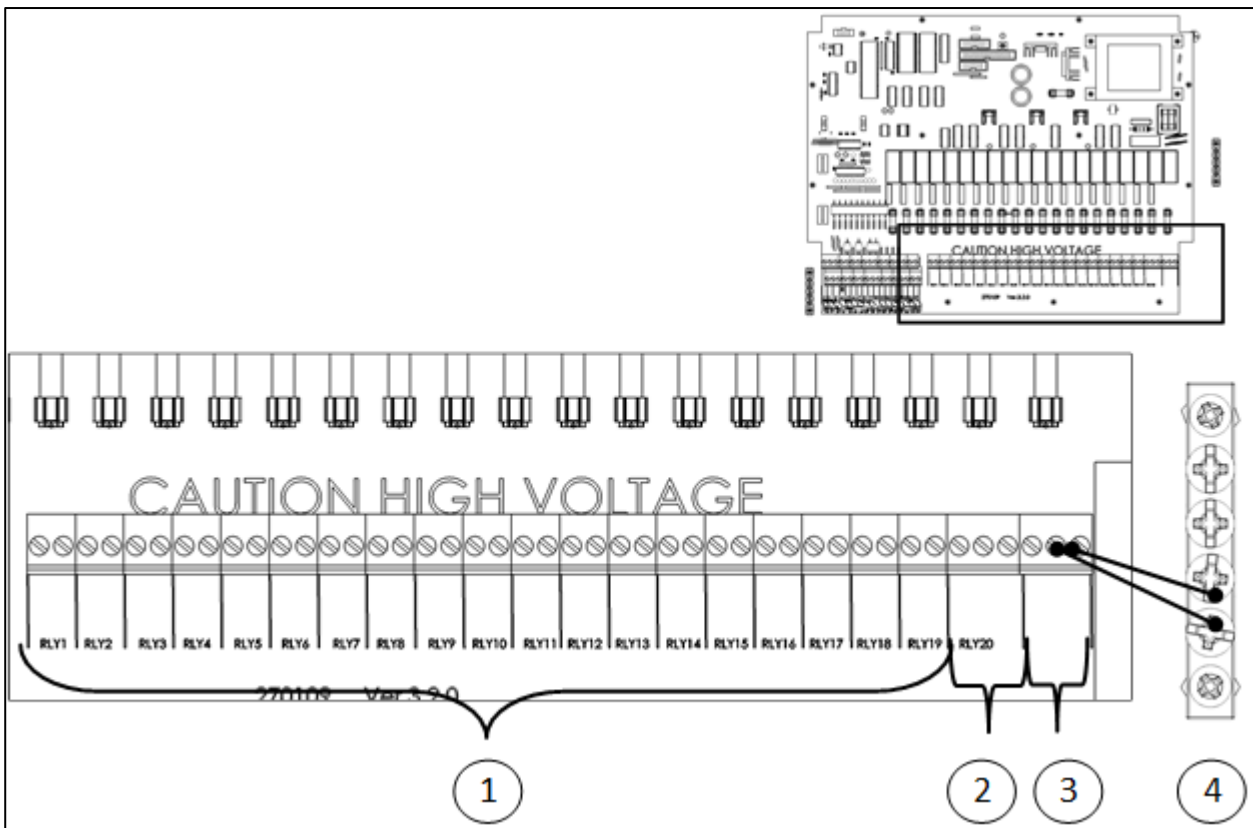
Figura 2: AC-2000 relés
