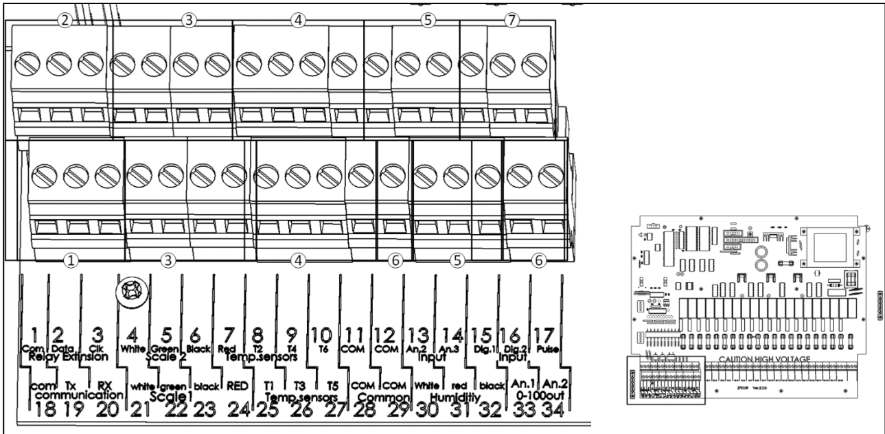
Figura 4: AC-2000 Plus terminales
