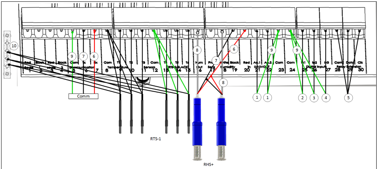
Figura 9: AC-2000 SE Cableado Eléctrico de Baja Tensión
