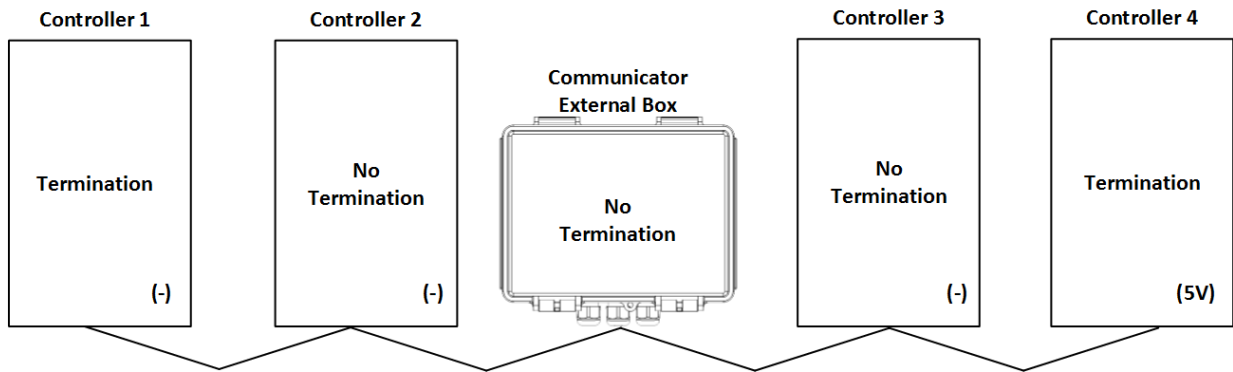
图 22: 控制器终端电阻
