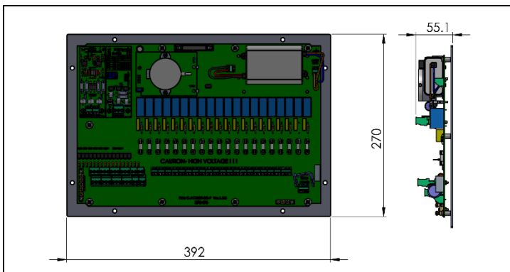
图 30: 基本尺寸
