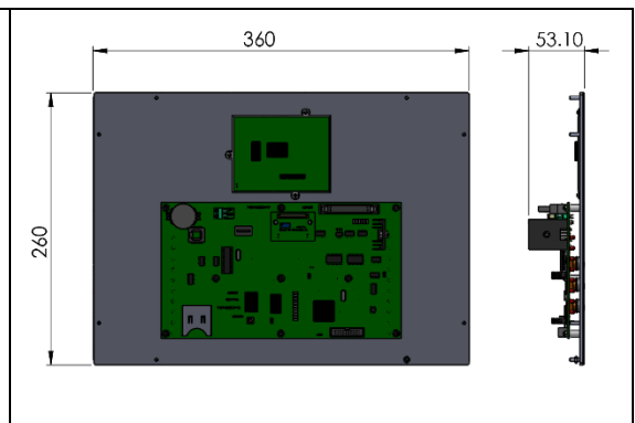
图 31: 封面尺寸
