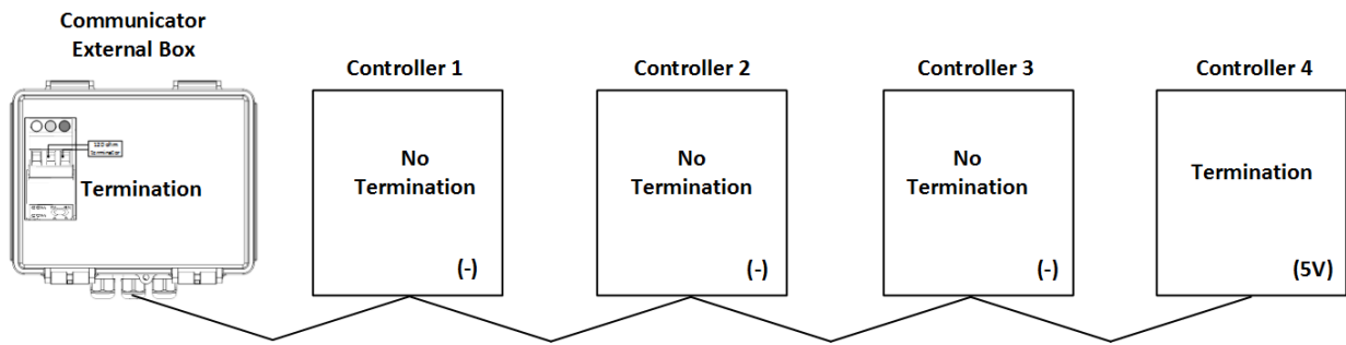
图 21: 外盒/控制器终端电阻
