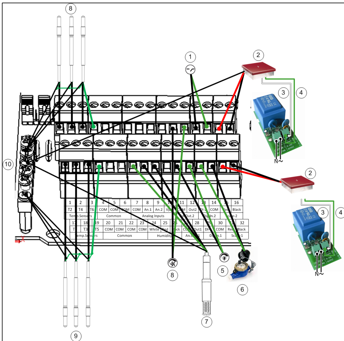
图 14: 低压模块接线
