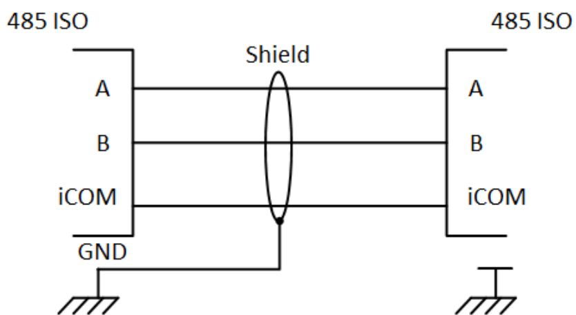
图 19: RS-485 (隔离)通讯卡至 MUX/通讯外盒接线
