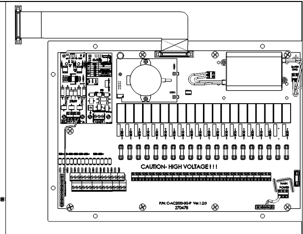
图 33: 卡板 / 扁平电缆
