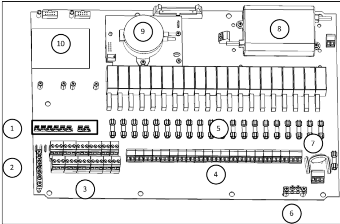
图 10: 主板布局
