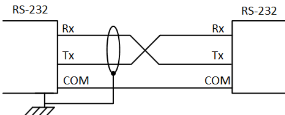
图 18: RS-232 通讯卡接线
