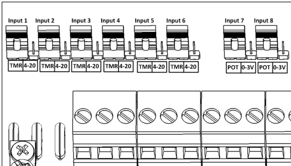
图 15: 跳线位置
