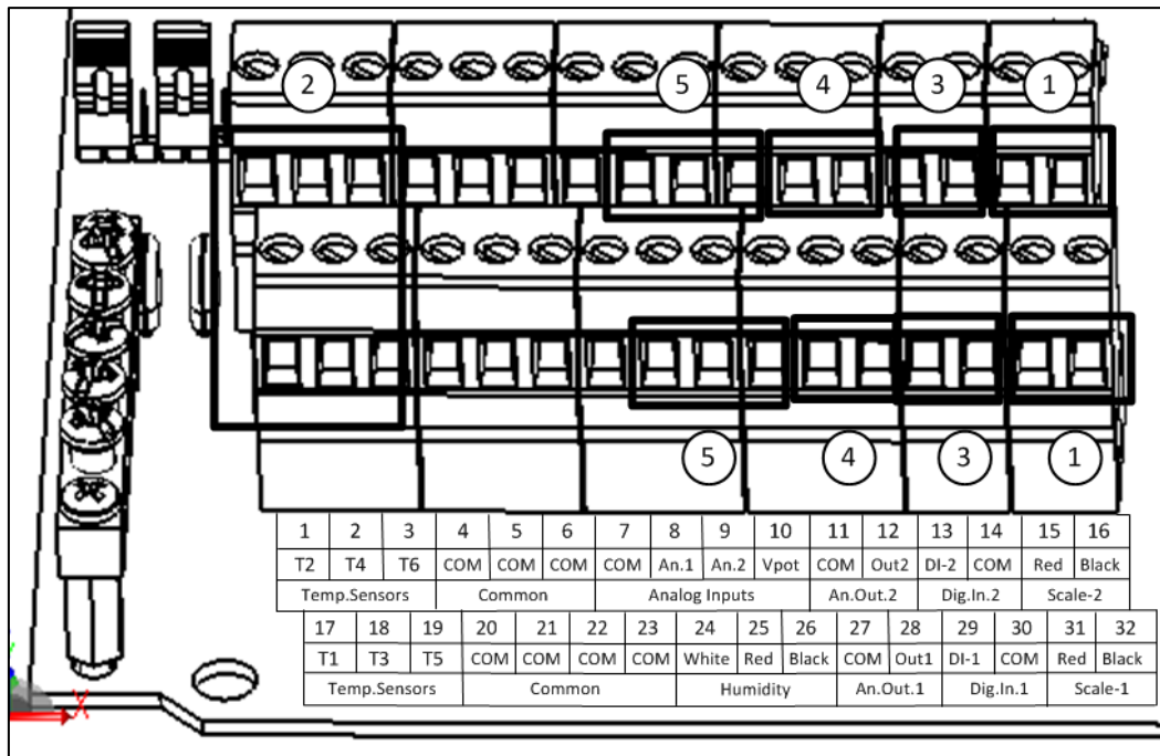
图 13: 端子
