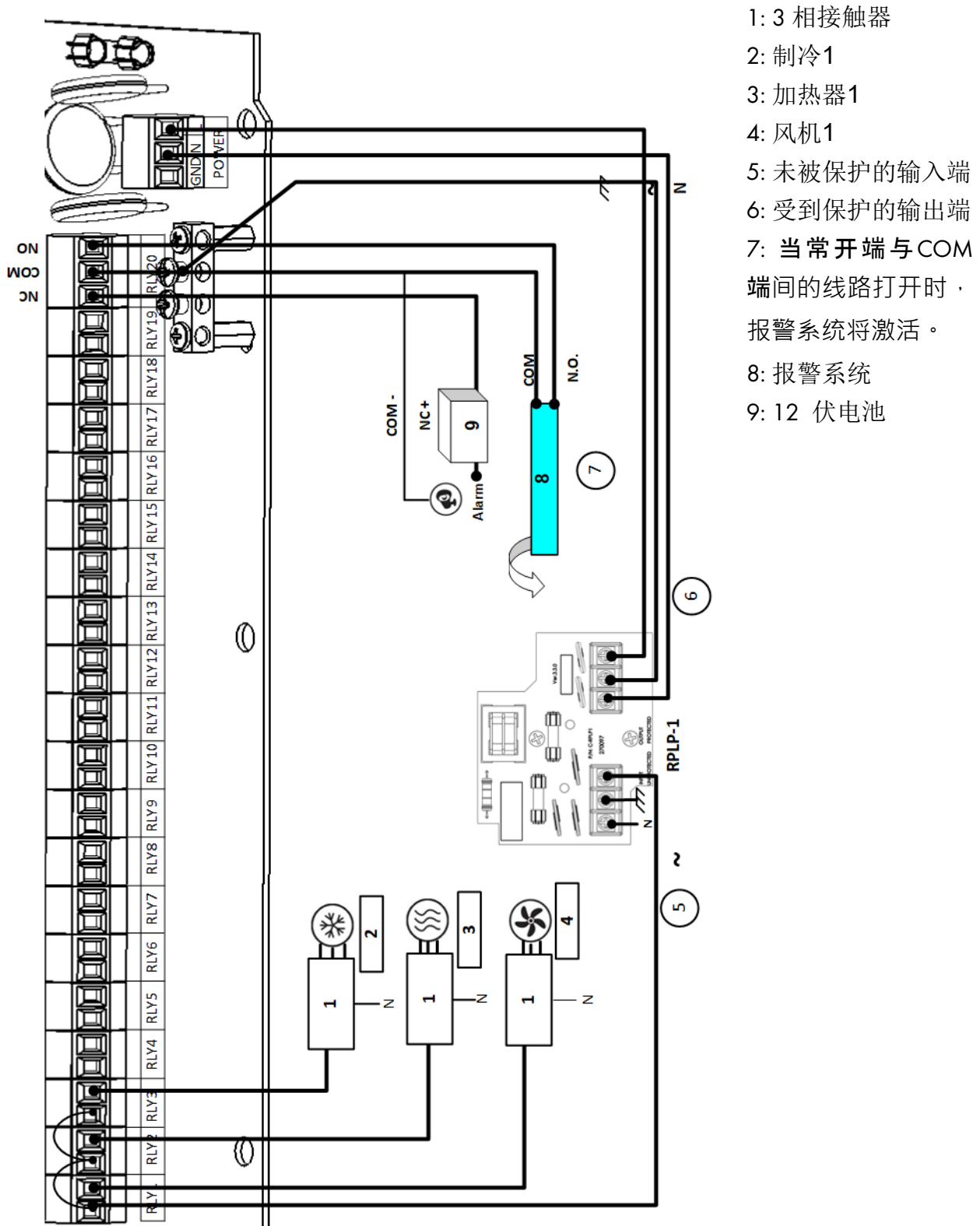
图 12: 压模块接线
