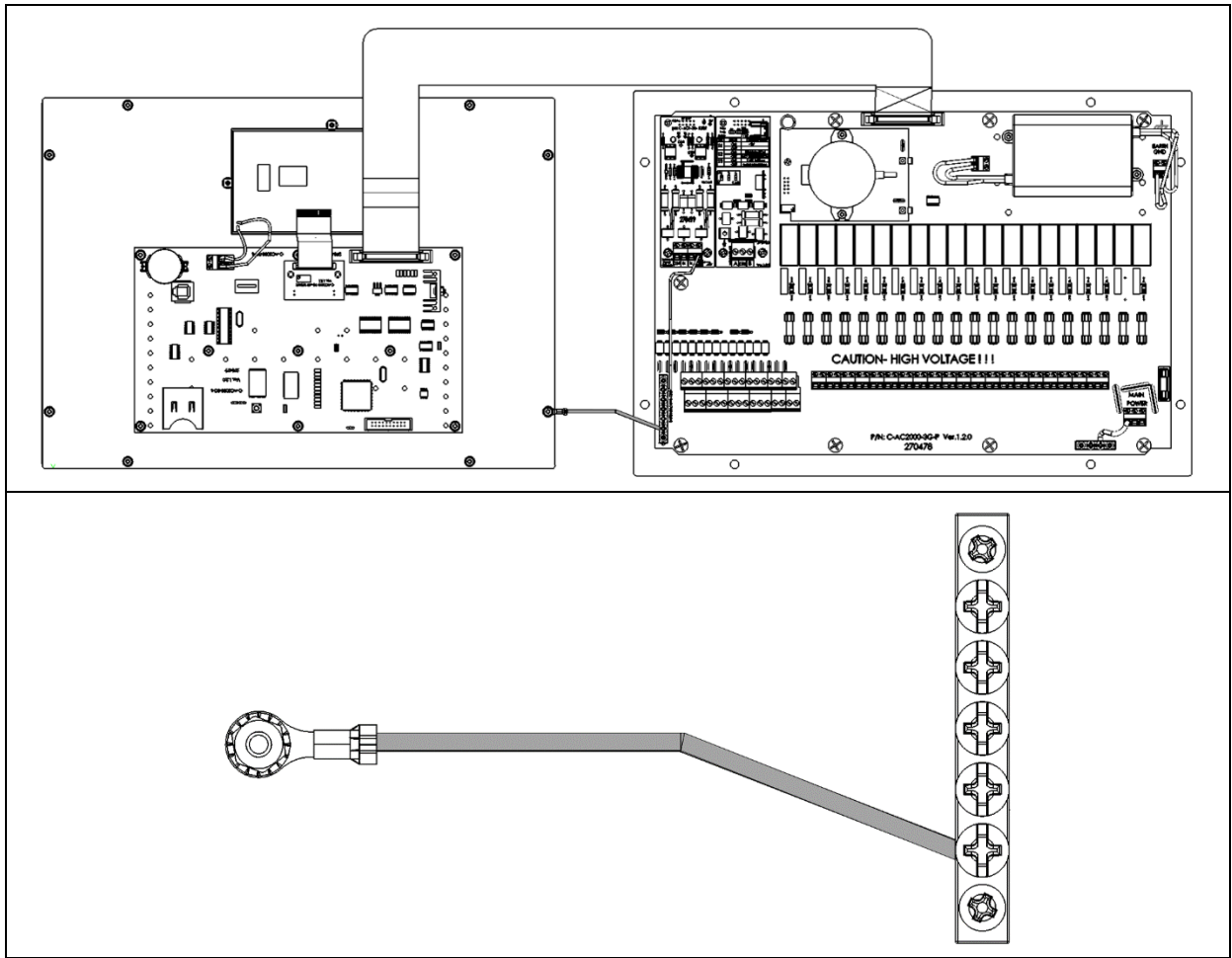
图 35: 接地电缆
