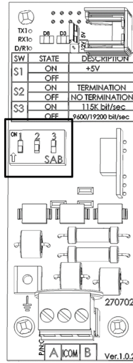
图 24: 隔离终端电阻禁用
