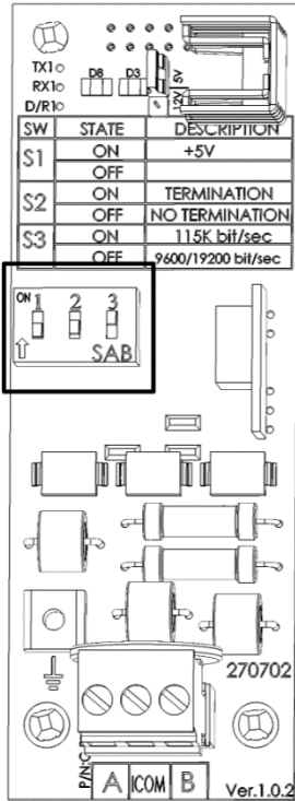
图 23: RS-485隔离终端电阻启用
