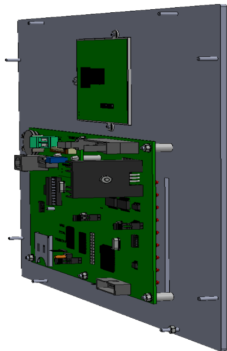
图 29: 盖板
