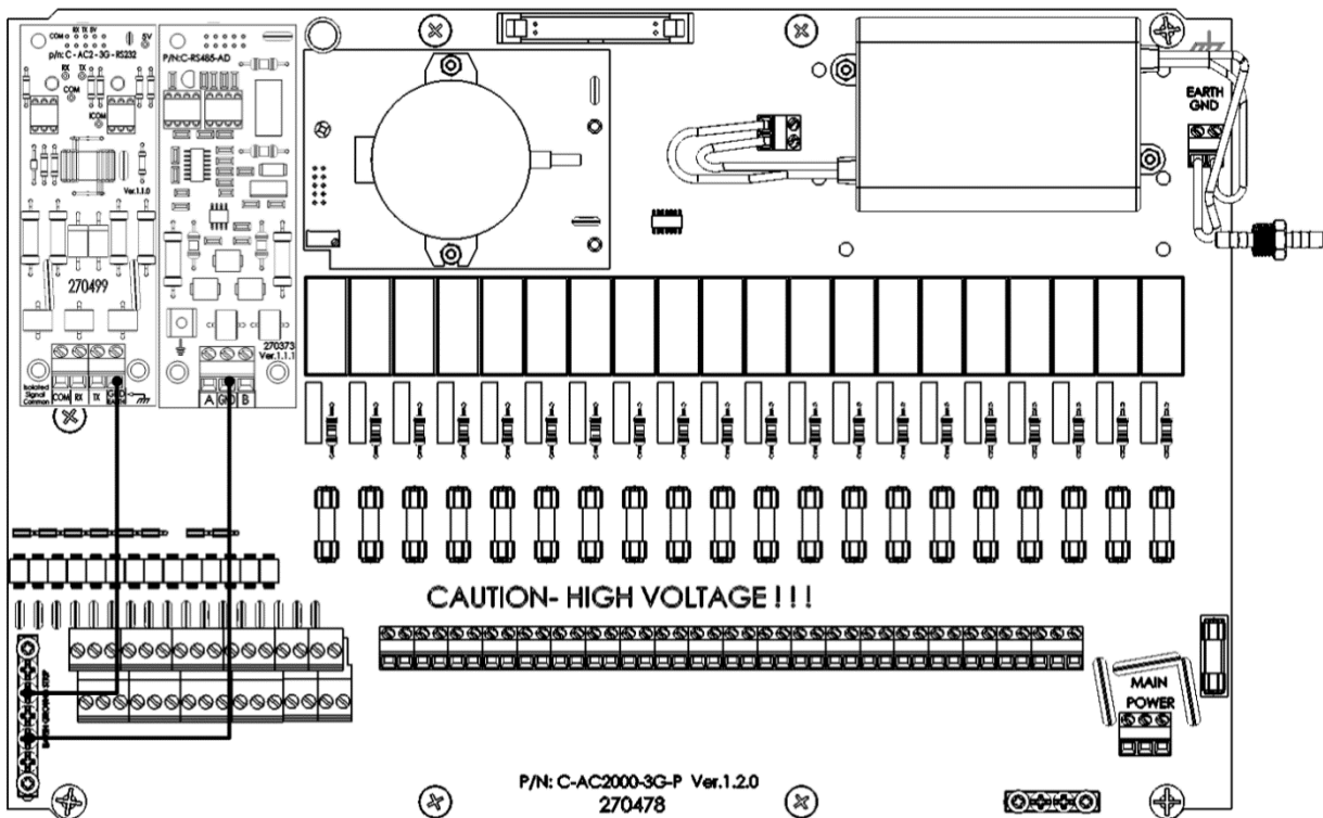
图 20: 通讯卡接地
