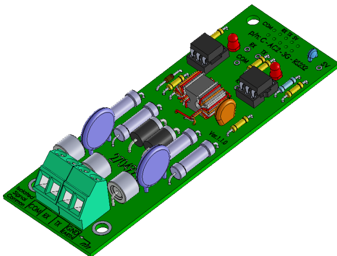
图 16: RNET-RS232卡 (P/N 904-99-00041)
