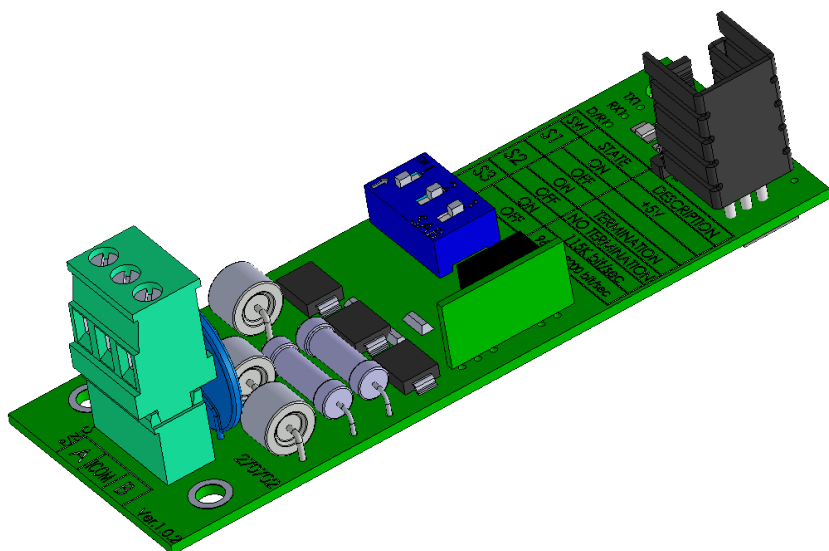
图 17: RNET RS-485隔离卡 (P/N: 905-99-00003)
